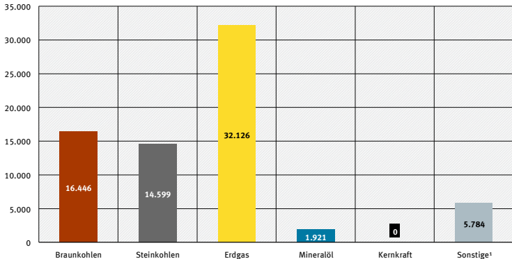
Elektrische Bruttoleistung in Megawatt
